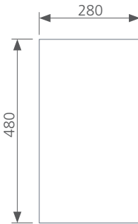
Cutout size / Medidas del corte para instalación
