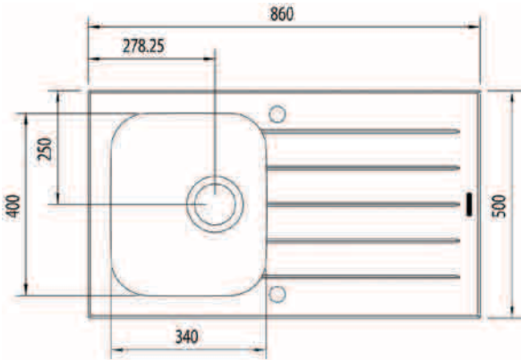
*Dimensions (mm) *Dimensiones (mm) Cutout size: 830 x 470 mm Medidas del corte para instalación: 830 x 470 mm
