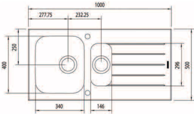
*Dimensions (mm) *Dimensiones (mm) Cutout size: 970 x 470 mm Medidas del corte para instalación: 970 x 470 mm
