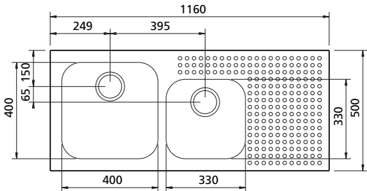
*Dimensions (mm) *Dimensiones (mm) Cutout size: 1140 x 480 mm Medidas del corte para instalación: 1140 x 480 mm
