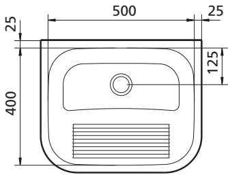
*Dimensions (mm) *Dimensiones (mm)
